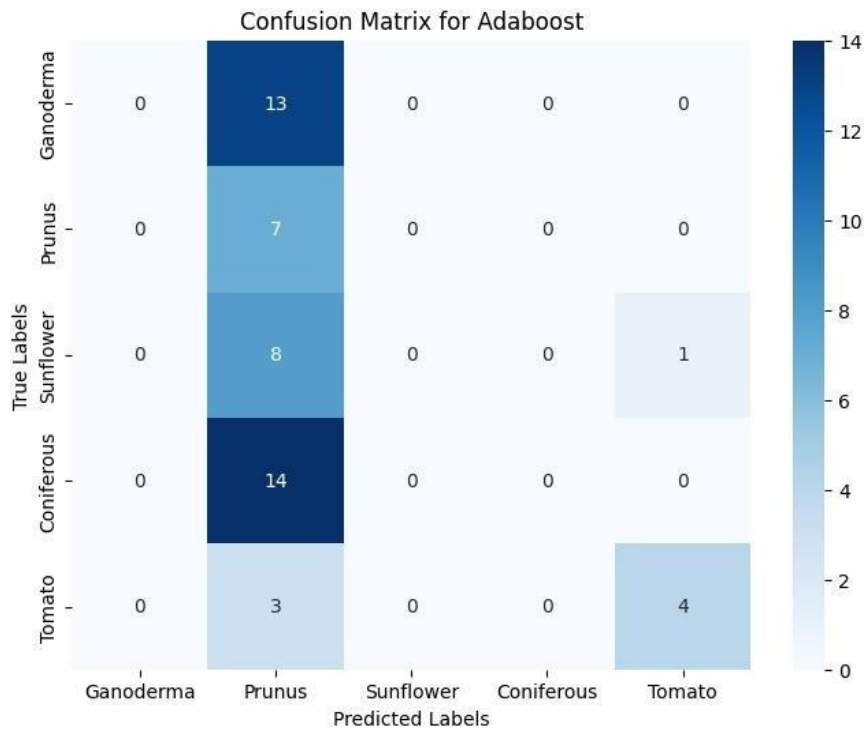
Fig 10. Adaboost Output
