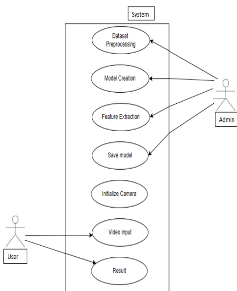
User-Case Diagram
