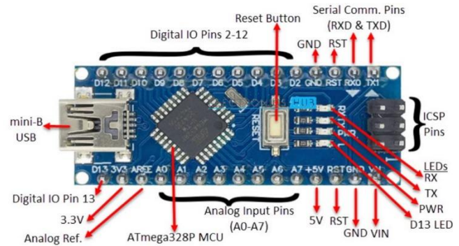
Fig. 3 Arduino Nano
