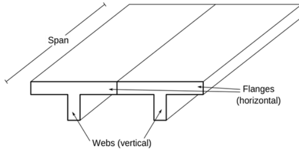
Fig 1. T-Beams
